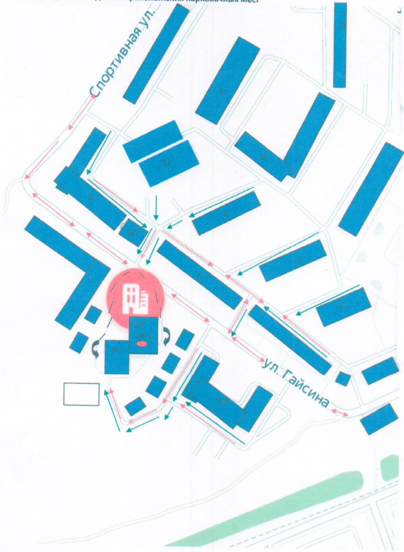
2. Схема организации дорожного движения в непосредственной близости от образовательного учреждения с размещением соответствующих технических средств организации дорожного движения, маршрутов движения детей и расположением парковочных мест
