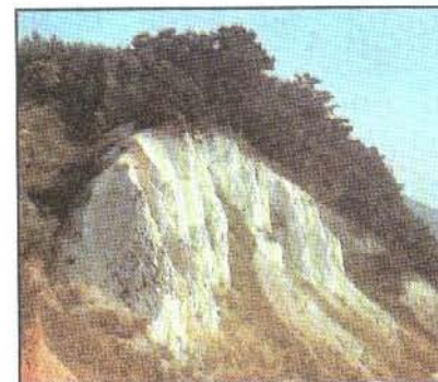
Залежи известняка
