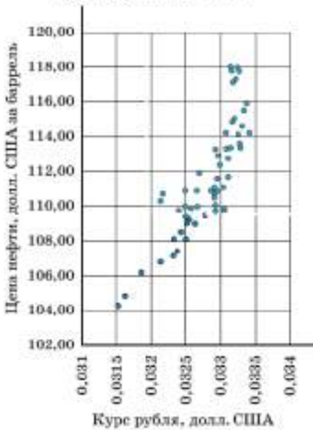
Диаграмма 32. Цена нефти — курс рубля, 2013 г.
