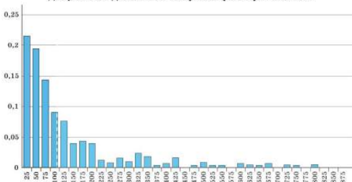
Диаграмма 24. Длительность телефонных разговоров. Шаг 25 с
