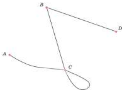
Рисунок 25. Граф с петлей в вершине С
