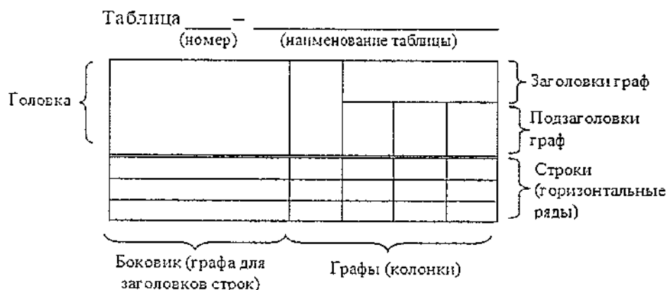
Рисунок 1 – Структура таблицы
