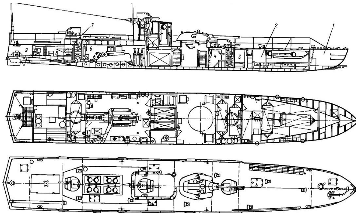
Рис. 5. Схемы общего расположения БКА по проекту 1125: прод. разрез, вид сверху, план. 1 - форпик; 2 - кубрик на 6 чел. , в котором выгорожена каюта командира; 3 - носовой пулеметный отсек; 4 - носовой боевой (подбашенный) отсек; 5 под боевой (ходовой) рубкой: по левому борту - радиорубка, в центре топливный отсек (бакн), по правому борту - коридор (здесь же унитаз); 6 моторное отделение; 7 - кормовой пулеметный отсек; 8 - хозотсек (камбуз); 9 - ахтерпик (румпельное отделение).
