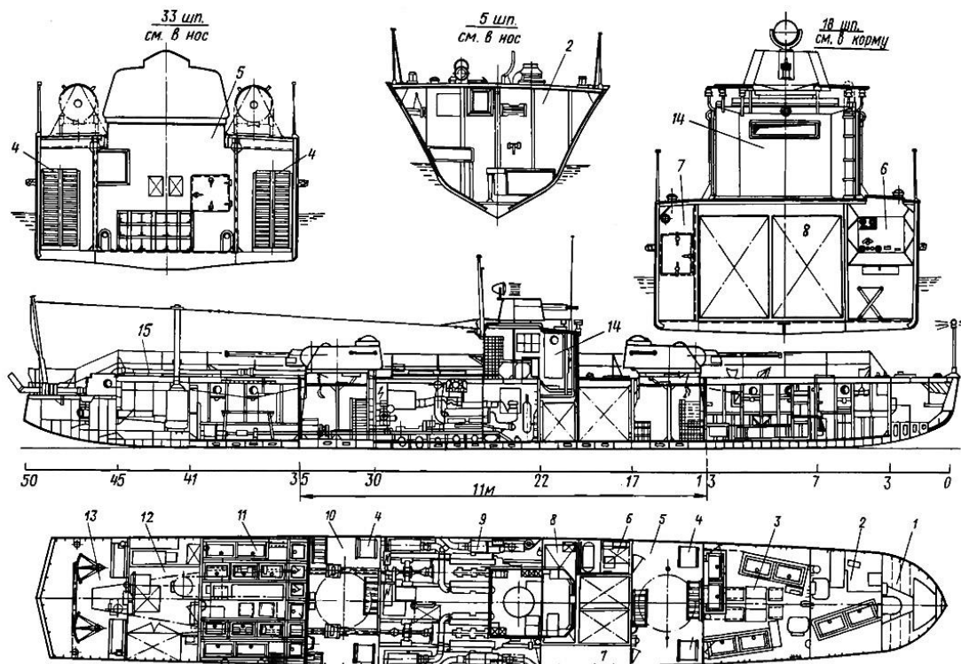
Рис. 2. Схемы общего расположения (прод. разрез, план и поперечные сечения) БКА по проекту 1124.
