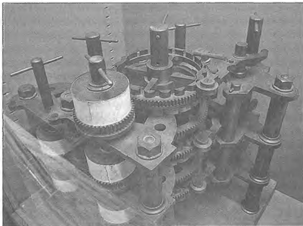
Рис. 3.1. Машина Бэббиджа
