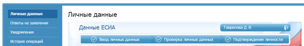
Рисунок 6. Данные ЕСИА.
