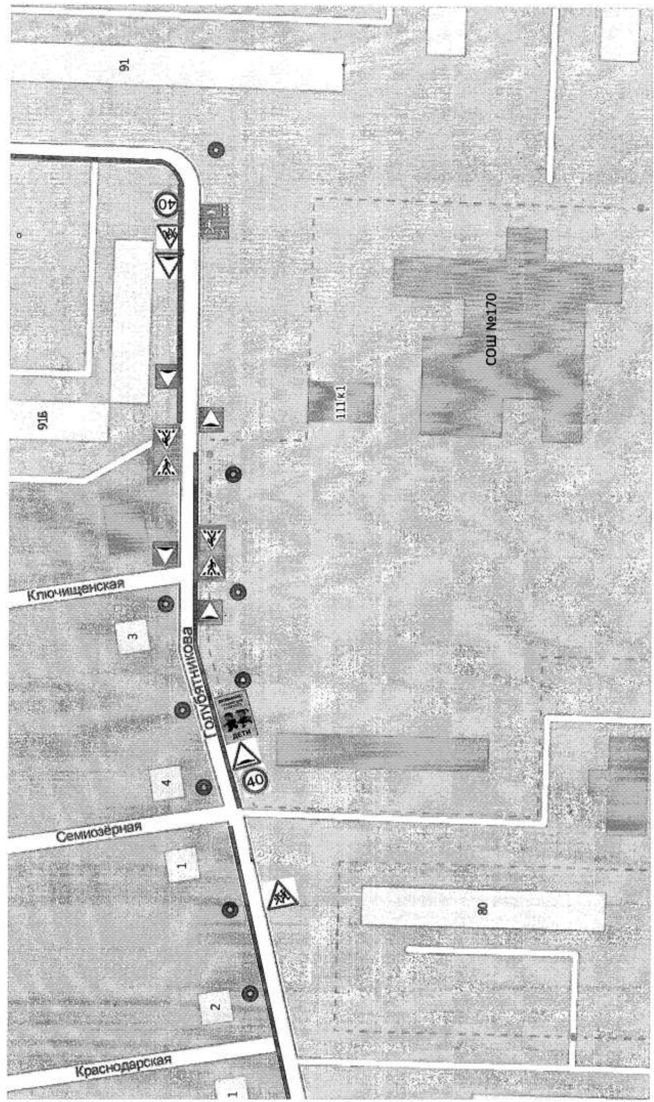
Схема организации дорожного движения в непосредственной близости от образовательного учреждения с размещением соответствующих технических средств организации дорожного движения, маршрутов движения детей и расположения парковочных мест
