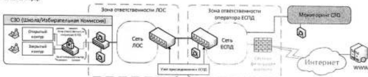
Рис.3 Схема подключения для услуги подключение к ЕСПД.
