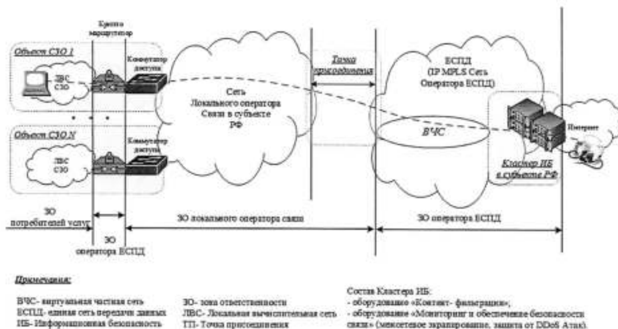
Рис. 5. Общая архитектура решений по контентной фильтрации.
