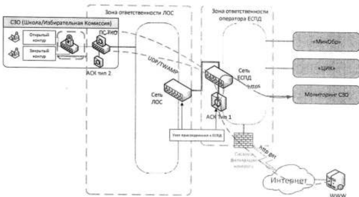
Рис.6 Общая типовая схема контроля качества услуг связи в открытом контуре узла СЗО «Школа/Избирательная комиссия»
