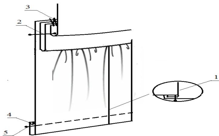
Рисунок 2 – Схема обработки рукава свитшота
